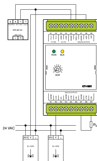
Zapojení 4 analogových výstupních kanálů
