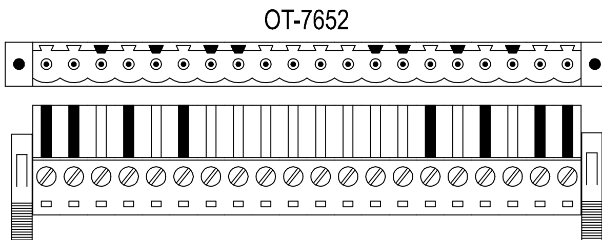
obr. 9.1 Kód konektoru modulu OT-7652
