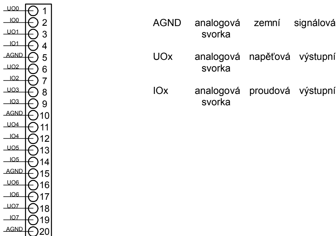
obr. 5.1 Zapojení svorkovnice modulu OT-7652
