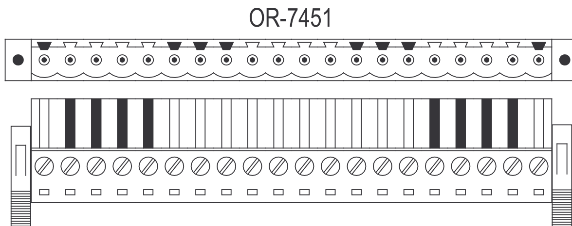
obr. 9.1 Kód konektoru modulu OR-7451
