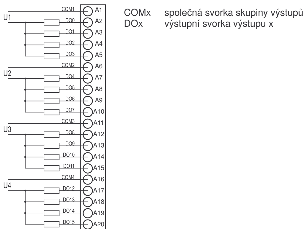
obr. 5.1 Zapojení konektoru modulu OR-7451
