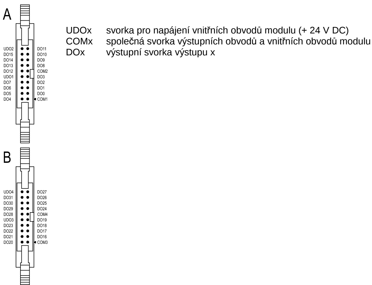
obr. 5.1 Zapojení konektorů modulu OS-7411
