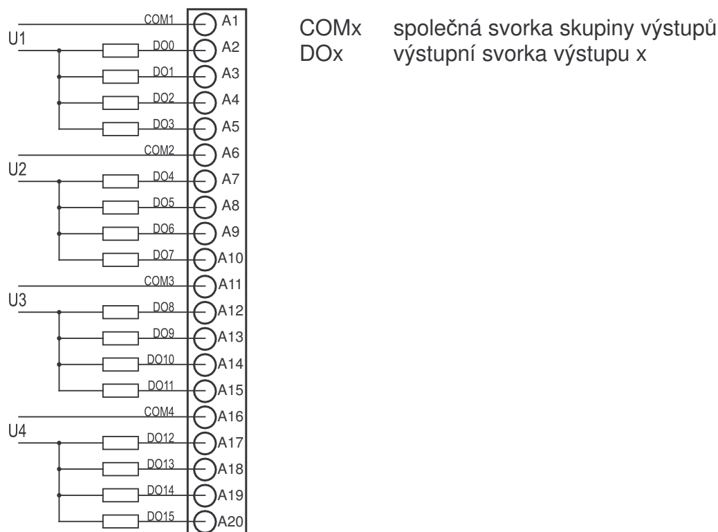
obr. 5.1 Zapojení konektoru modulu OS-7405
