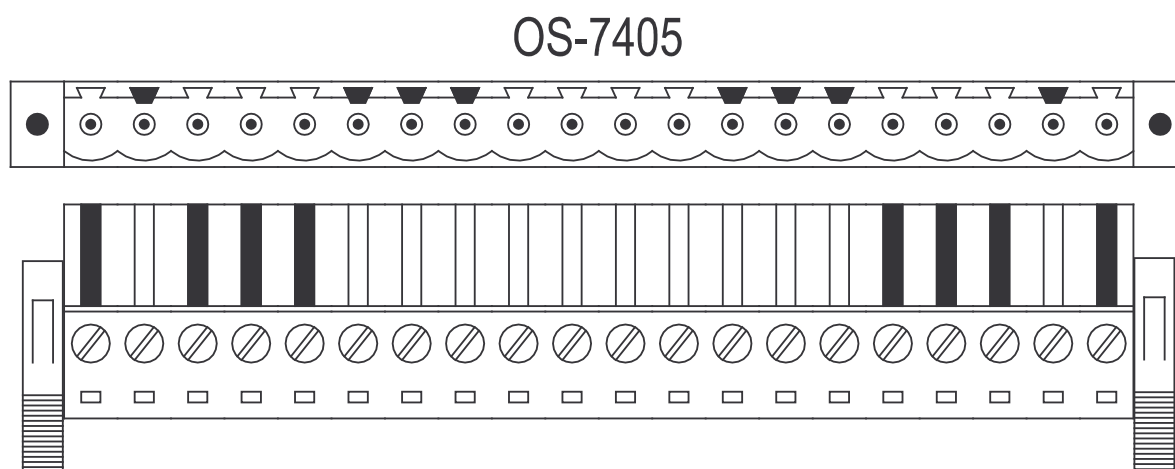
obr. 9.1 Kód konektoru modulu OS-7405
