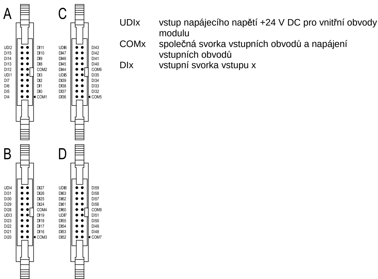
obr. 5.1 Zapojení konektoru modulu IB-7310
