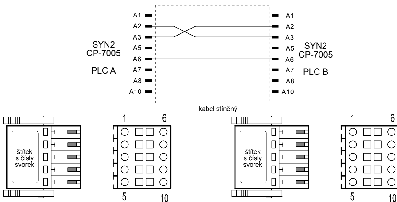
obr. 5.1 Vzájemné propojení rozhraní SYN2 dvou CP-7005 (redundantní zapojení)
