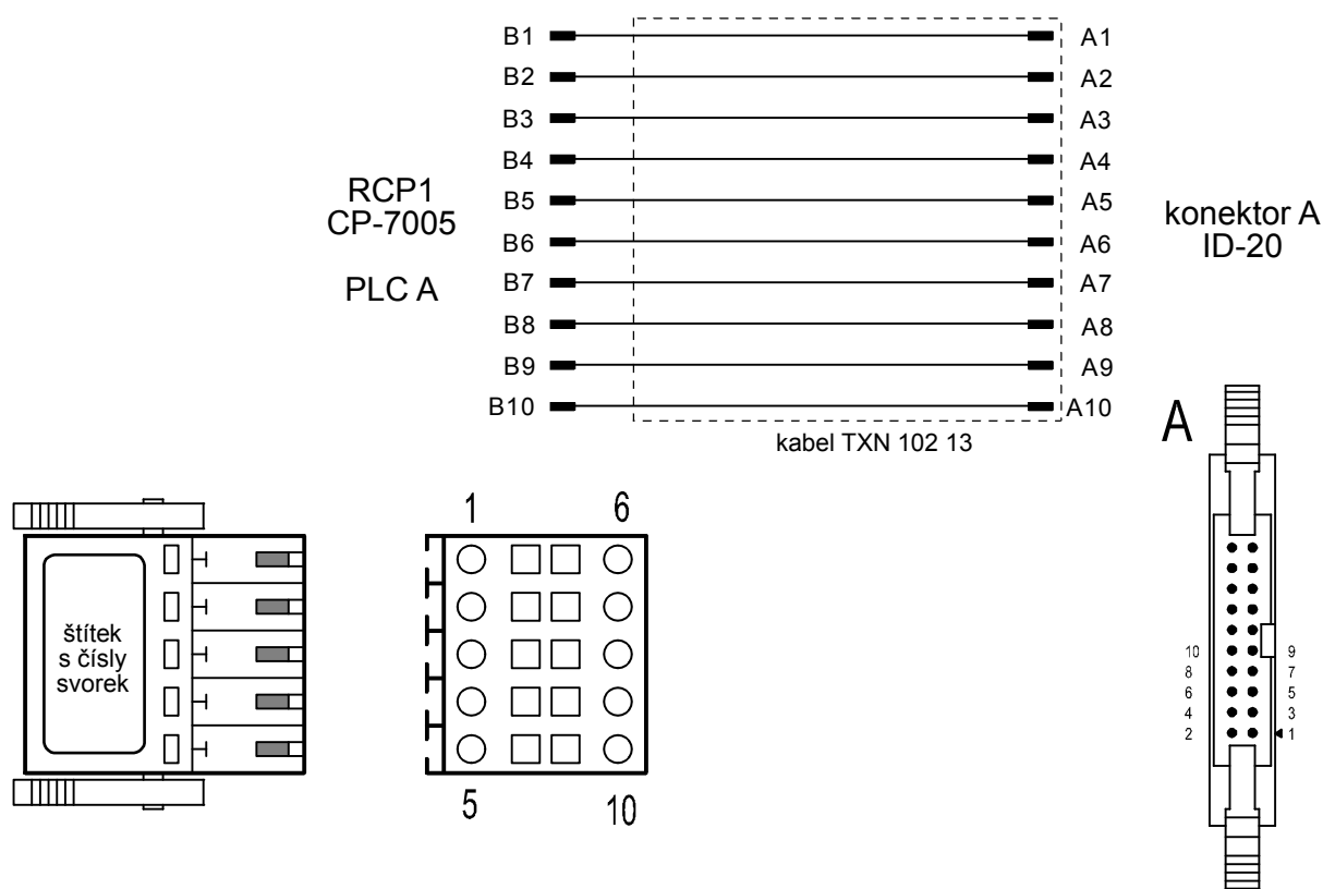
obr. 5.2 Propojení rozhraní RCP1 CP-7005 (PLC A) a konektoru A modulu ID-20
