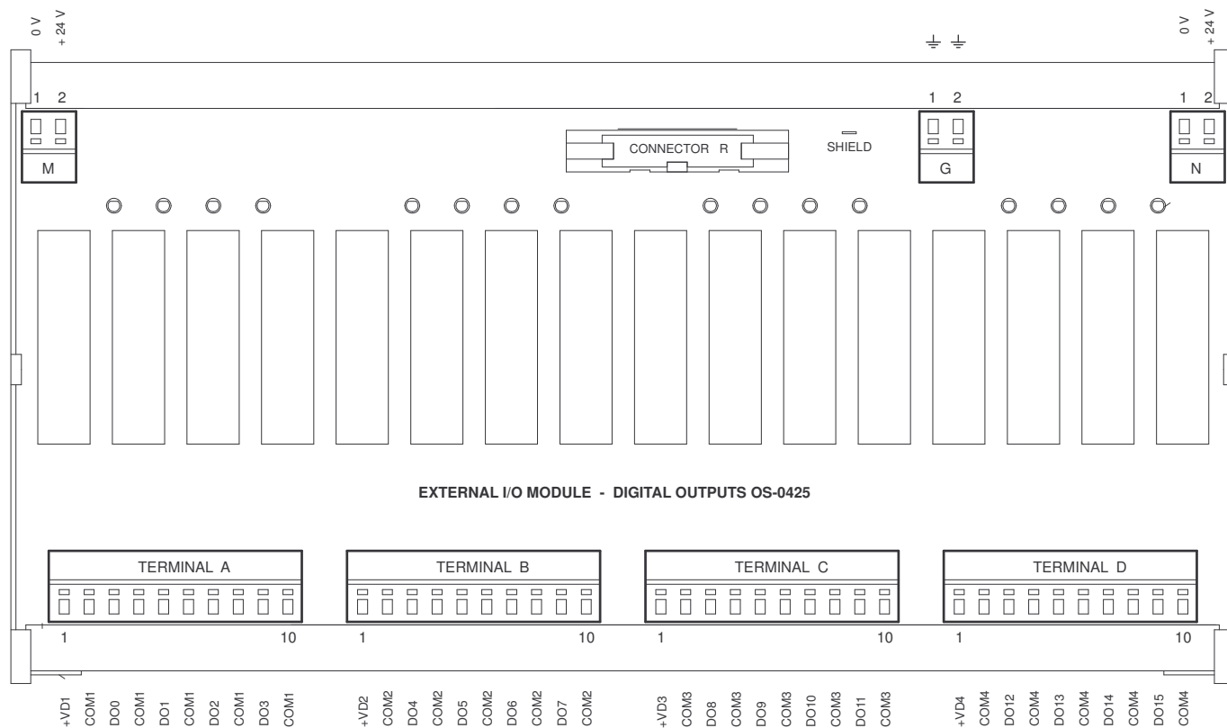
obr. 5.1 Zapojení konektoru modulu OS-0425
