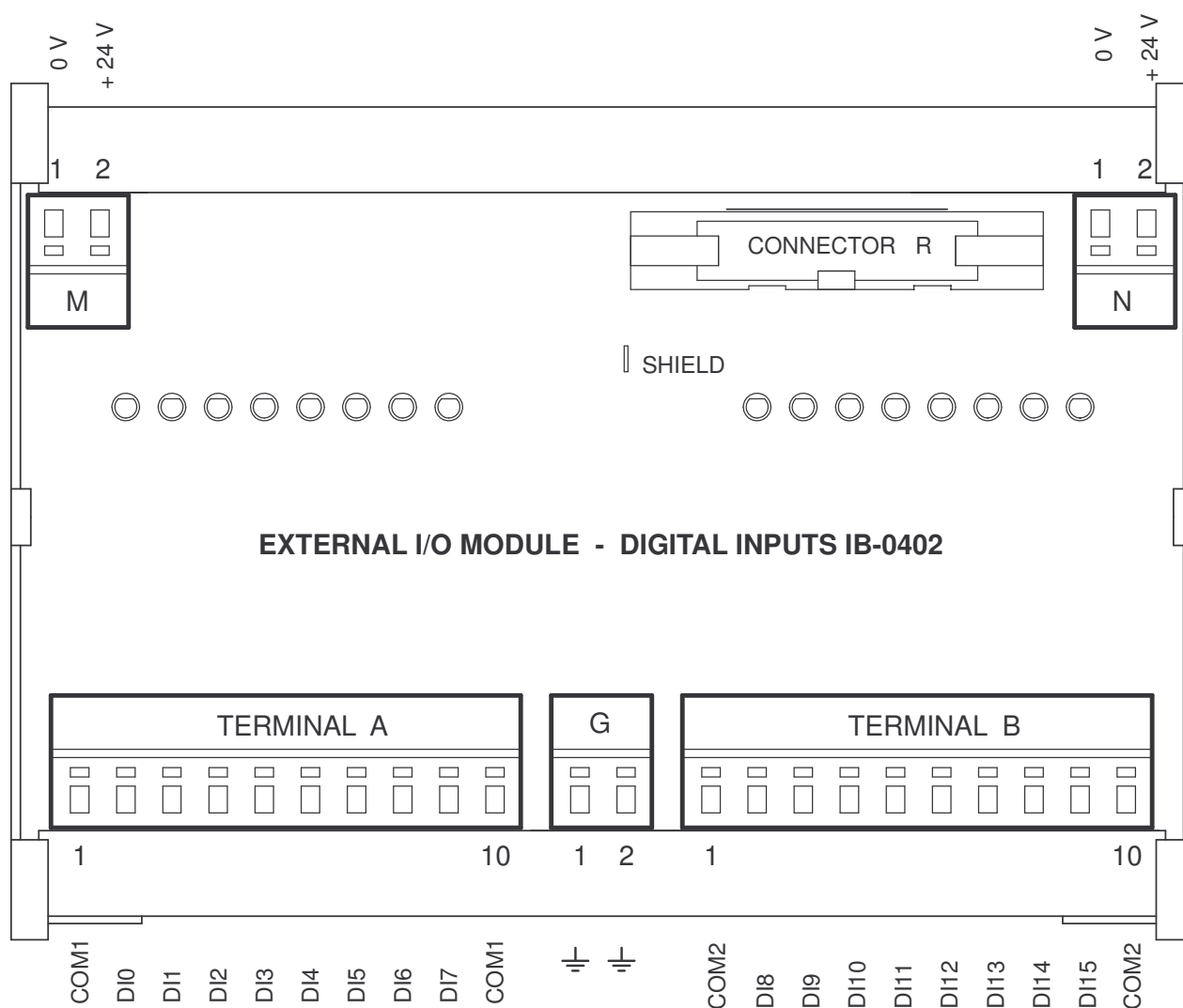
obr. 5.1 Zapojení konektoru modulu IB-0402
