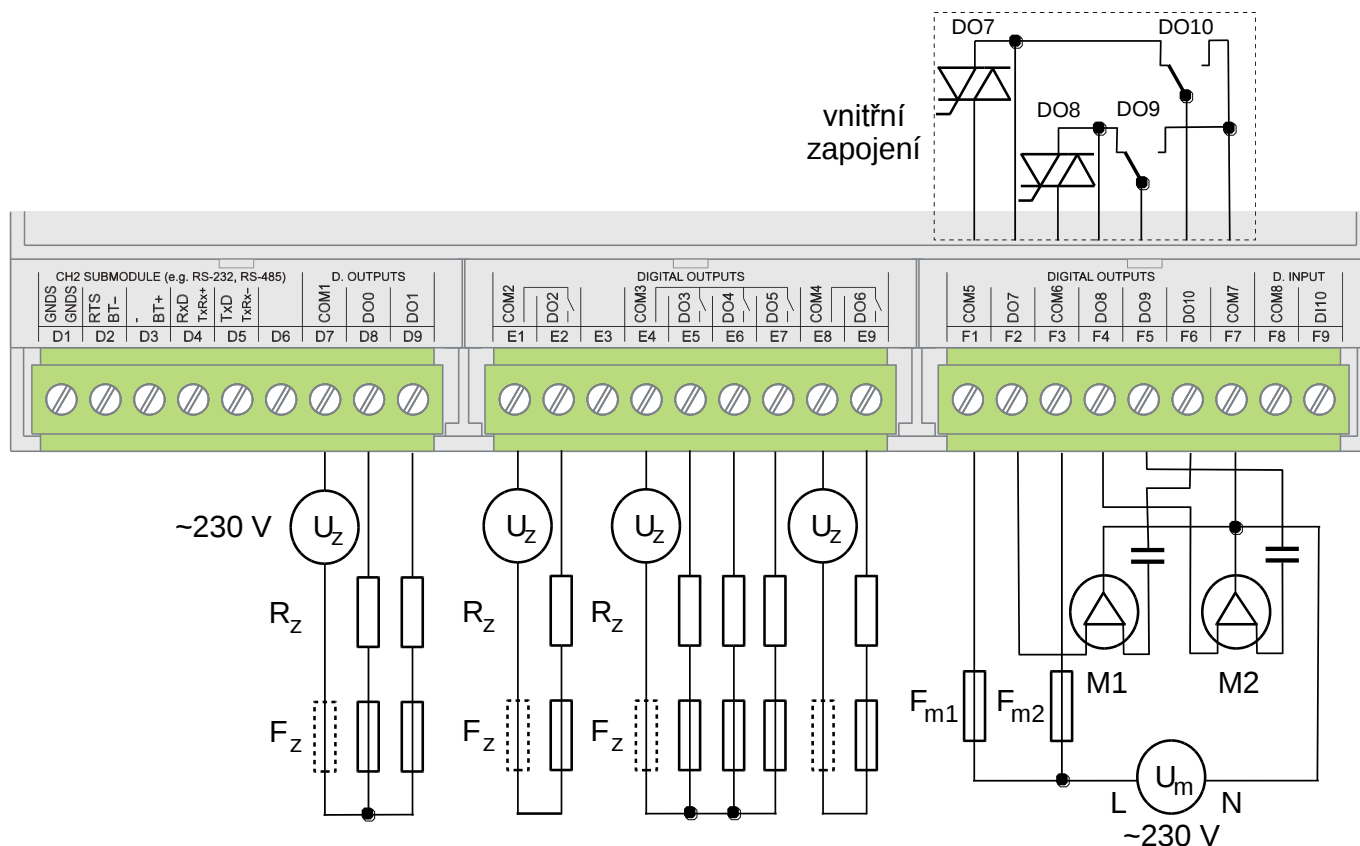
Obr.4.2 Typický příklad připojení zátěží k binárním výstupům základního modulu CP-10x8 (na výstupech DO7 - DO10 naznačeno připojení AC motorů)
