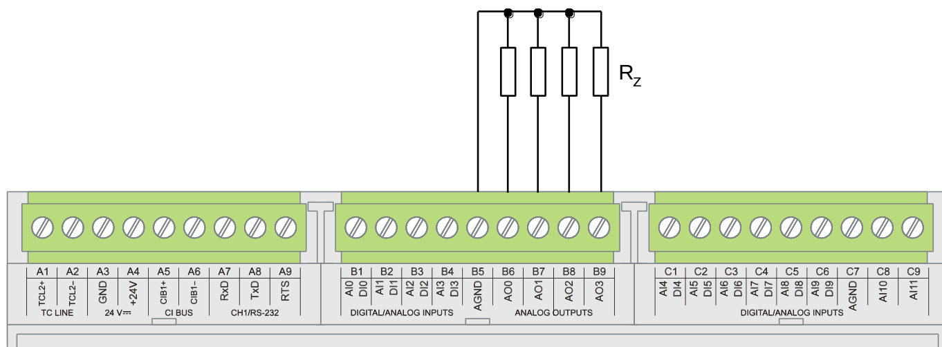
Obr.4.5 Typický příklad připojení zátěží k analogovým výstupům základního modulu CP-10x8
