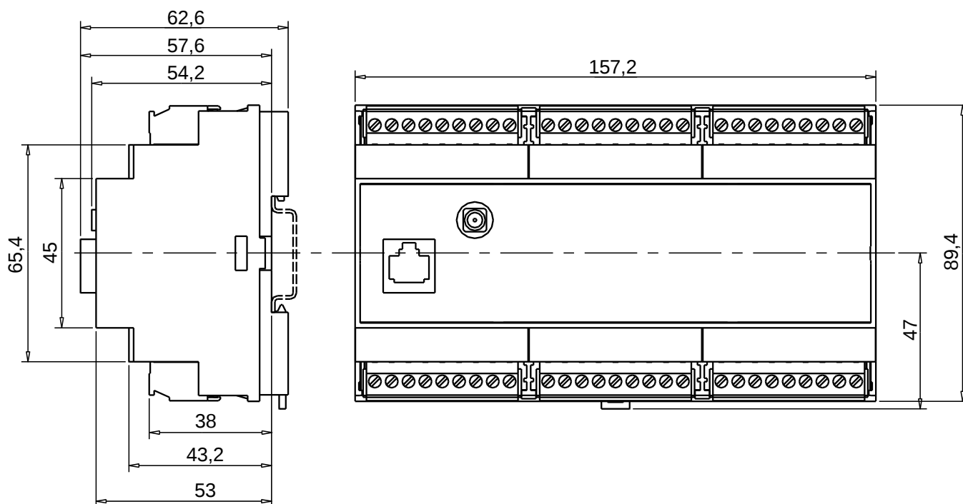
Obr.2.1 Rozměry základních modulů CP-10x8
