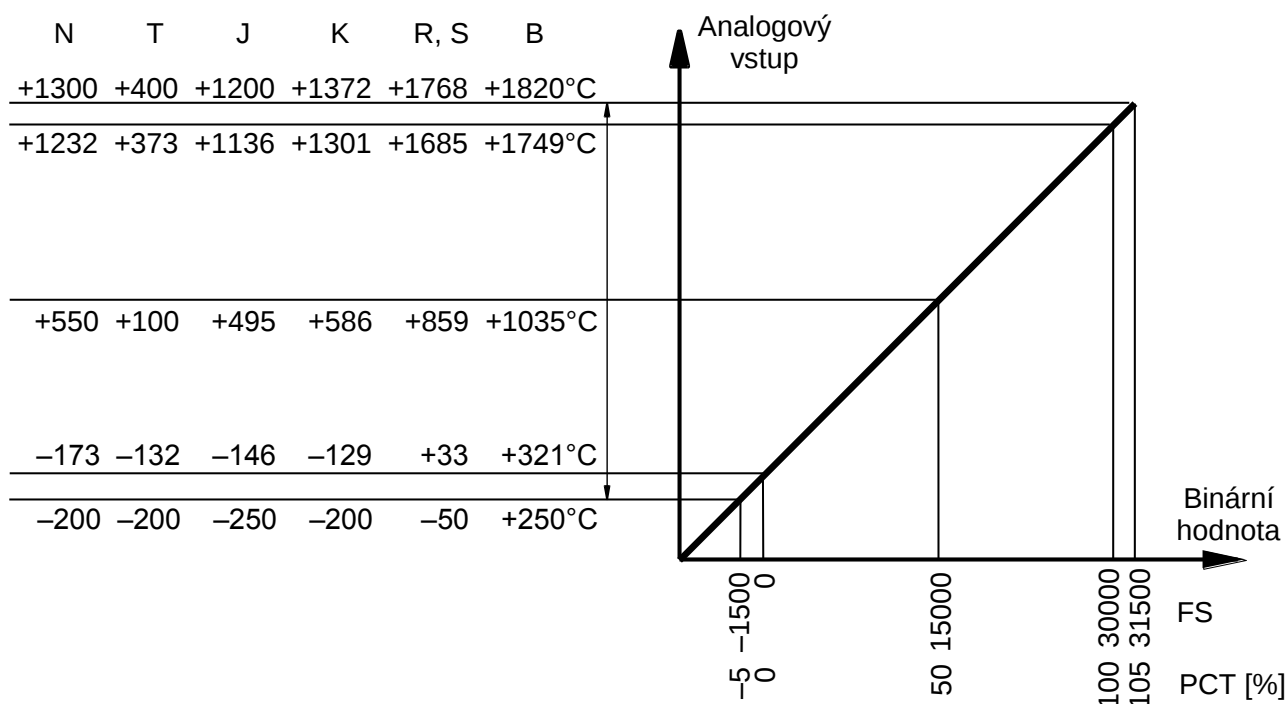
Obr.4.19 Rozsah analogových vstupů AI10 a AI11 modulu CP-10x8 pro termočláanky
