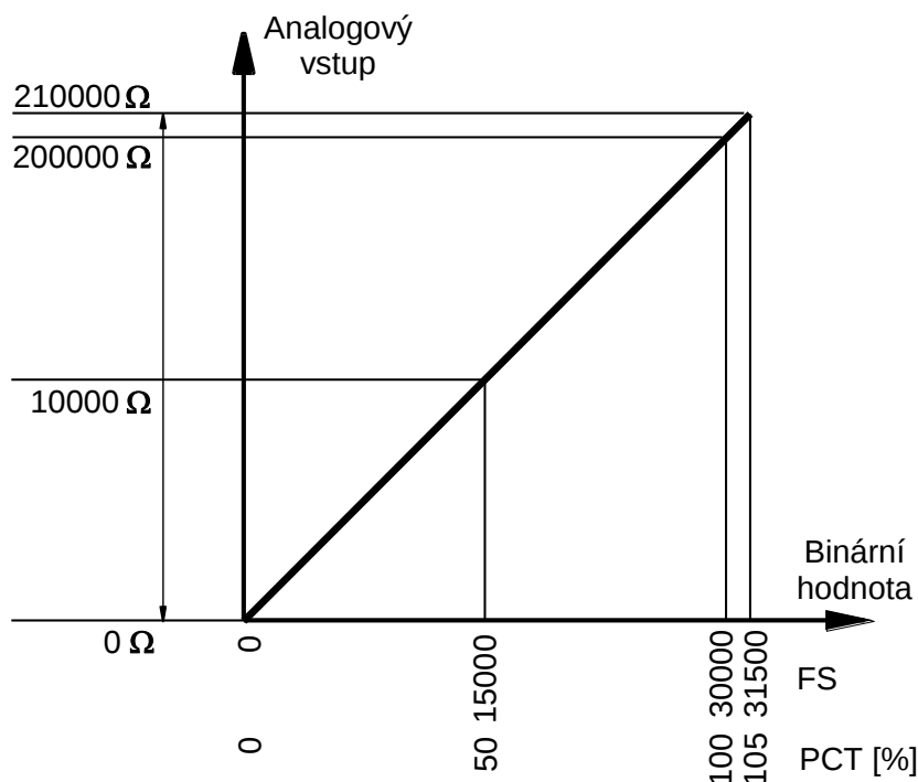
Obr.4.15 Odporový rozsah do 200 k \Omega analogových vstupů AI4 - AI9 modulu CP-10x8
