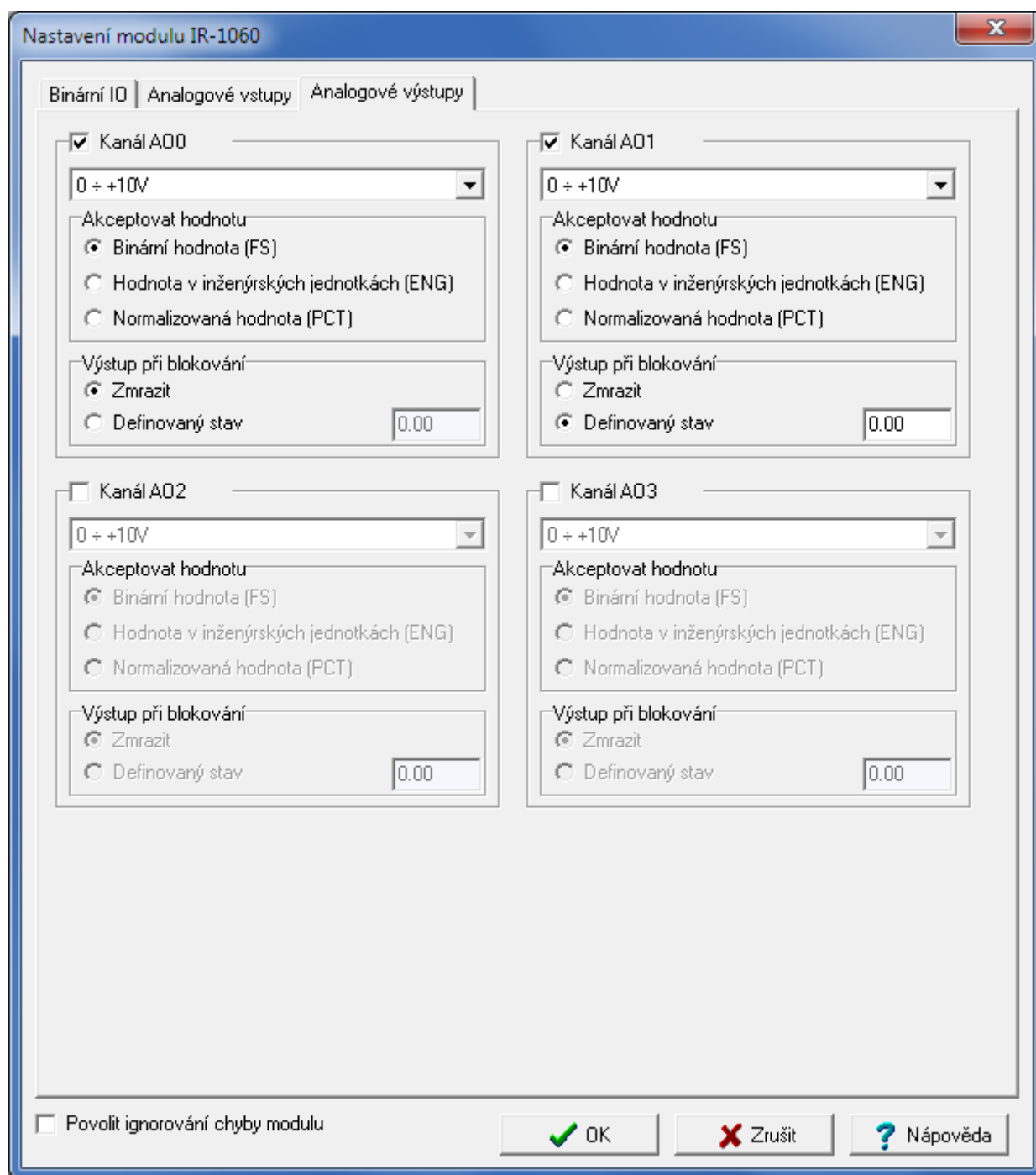
Obr.4.21 Konfigurace analogových výstupů
