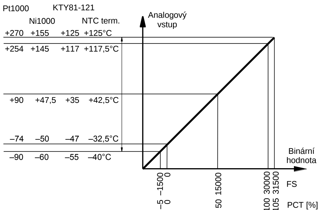
Obr.4.13 Rozsah analogových vstupů AI0 - AI9 modulu CP-10x8 pro odporová čidla Pt1000, Ni1000, KTY81-121 a NTC termistory (NTC termistory lze připojit jen ke vstupům AI4 - AI9)
