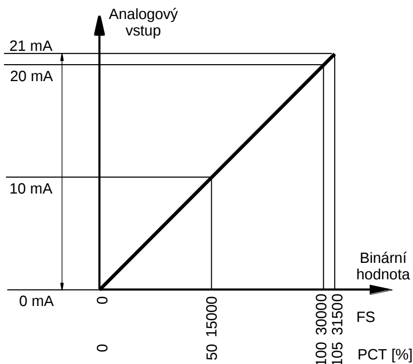
Obr.4.11 Proudový rozsah 0 až 20 mA analogových vstupů AI4 - AI9 modulu CP-10x8
