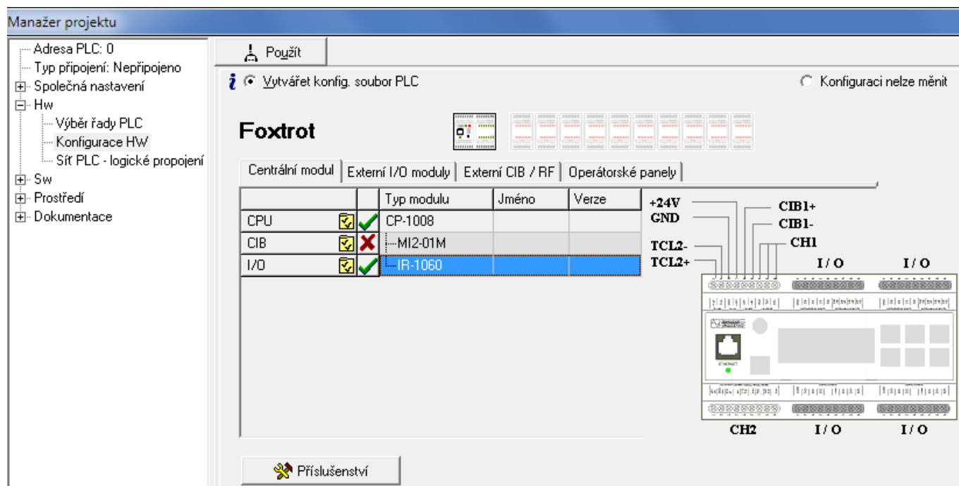
Obr.4.7 Konfigurace základního modulu CP-1008
