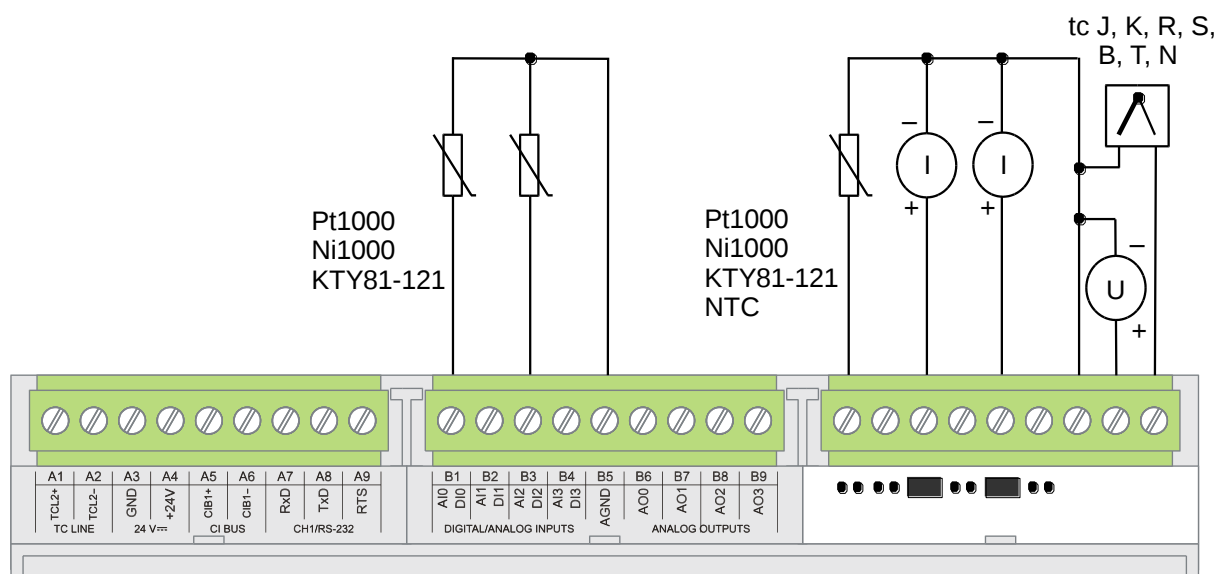
Obr.4.4 Typický příklad připojení signálů k analogovým vstupům základního modulu CP-10x8 (jednotlivé druhy signálů jsou připojitelné k analogovým vstupům podle tab.4.6 a tab.4.7)
