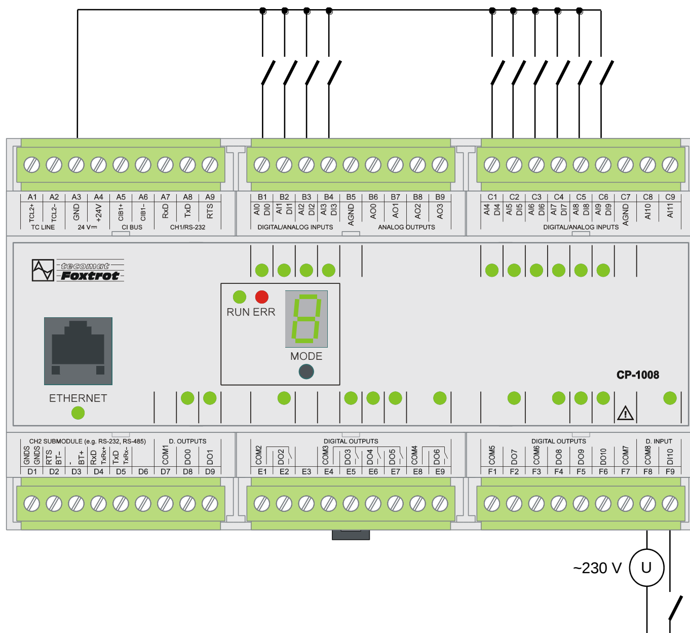
Obr.4.1 Typický příklad připojení spínačů k binárním vstupům základního modulu CP-10x8
