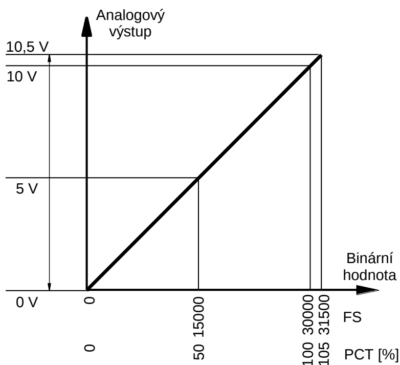
Obr.4.22 Rozsah analogových výstupů modulu CP-10x8
