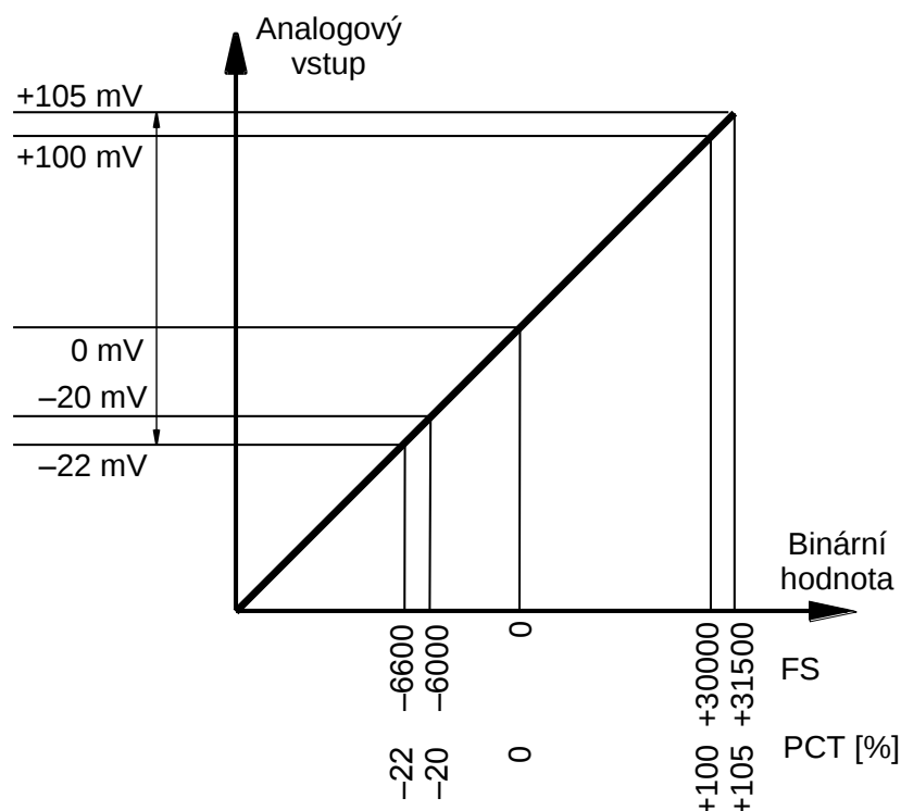
Obr.4.17 Napěťový rozsah -0,02 až +0,1 V analogových vstupů AI10 a AI11 modulu CP-10x8
