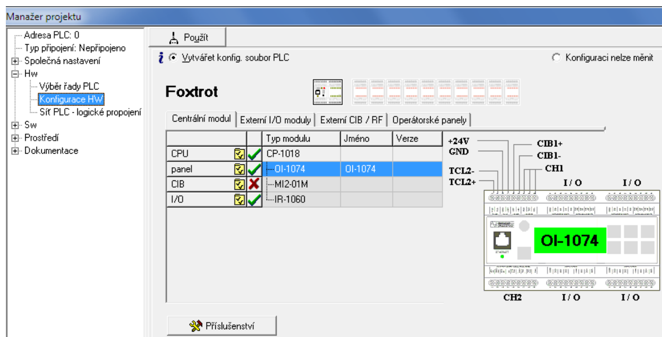
Obr.5.2 Konfigurace základního modulu CP-1014
