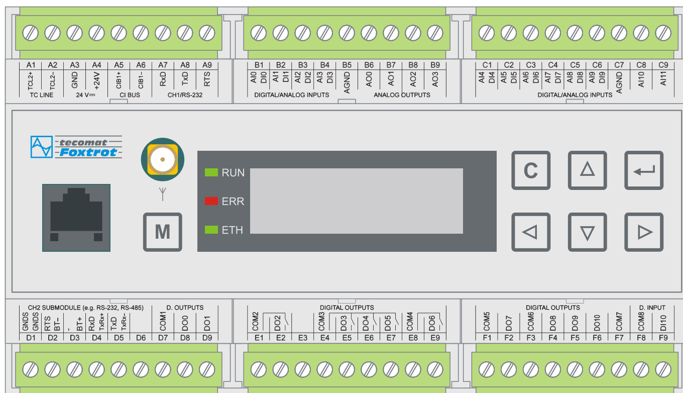
Obr.2.5 Základní modul CP-1038
