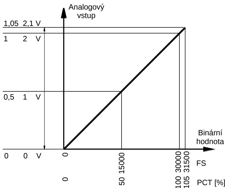
Obr.4.16 Napěťové rozsahy do 1 V a do 2 V analogových vstupů AI10 a AI11 modulu CP-10x8
