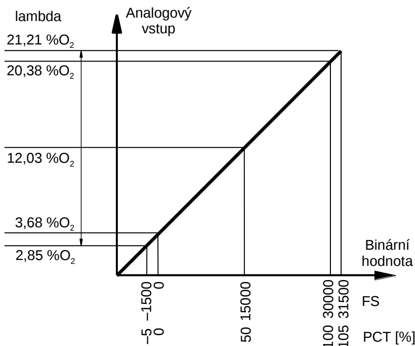
Obr.4.20 Rozsah analogových vstupů AI10 a AI11 modulu CP-10x8 pro lambda sondu
