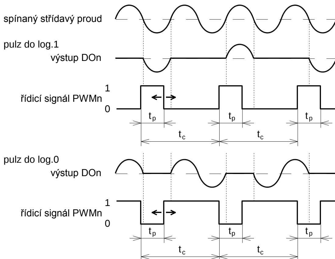
Obr.4.9 Výstup v režimu pulzně šířkové modulace PWM t_p - šířka pulzu, t_c = perioda
