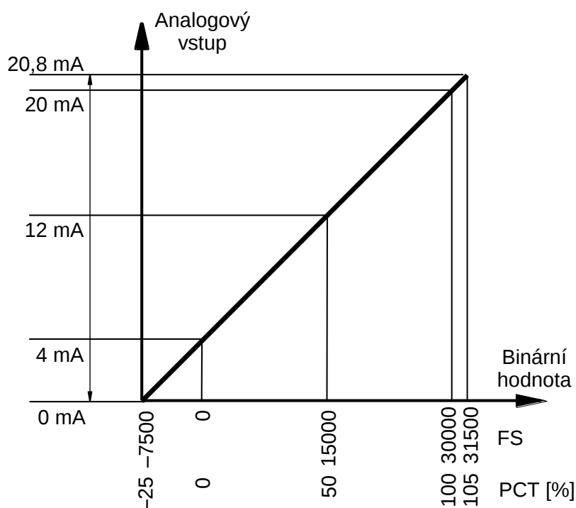
Obr.4.12 Proudový rozsah 4 až 20 mA analogových vstupů AI4 - AI9 modulu CP-10x8
