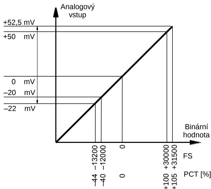
Obr.4.18 Napěťový rozsah -0,02 až +0,05 V analogových vstupů AI10 a AI11 modulu CP-10x8
