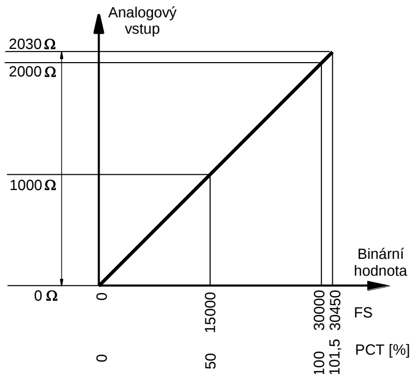
Obr.4.14 Odporový rozsah do 2000 \Omega analogových vstupů AI0 - AI9 modulu CP-10x8 (rozsah je v oblasti nad nominální hodnotou zkrácen z důvodu fyzického omezení rozsahu vstupů)
