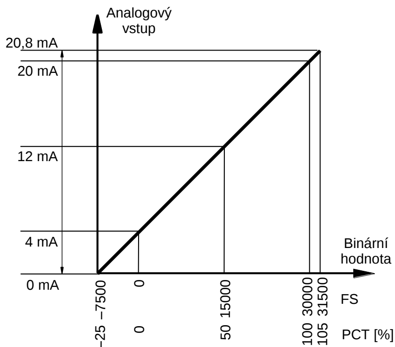
Obr.4.12 Proudový rozsah 4 až 20 mA analogových vstupů modulů CP-10x5
