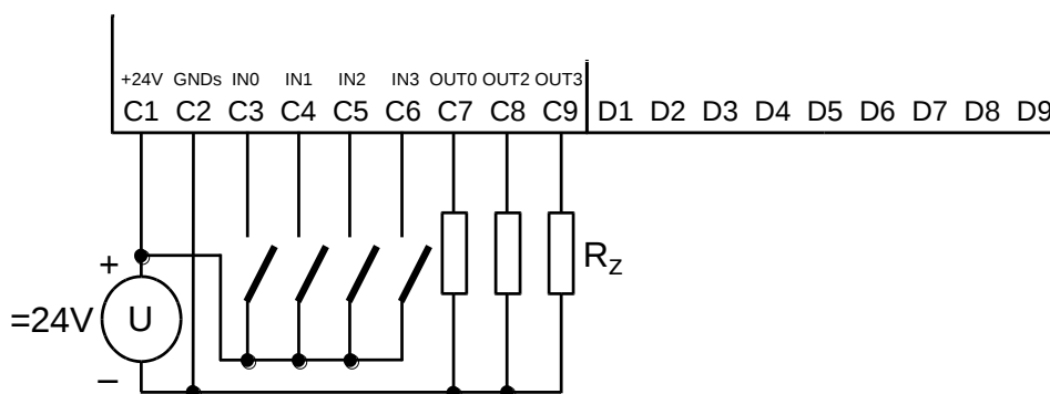
Obr.3.3 Typický příklad připojení spínačů a zátěží k základnímu modulu při osazeném submodule PX-7812 na kanálu CH2
