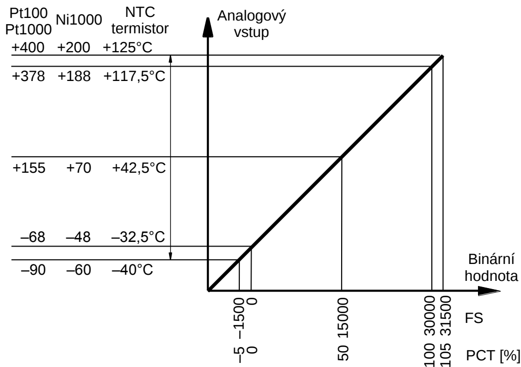
Obr.4.13 Rozsah analogových vstupů modulů CP-10x5 pro odporová čidla Pt100, Pt1000, Ni1000 a NTC termistory
