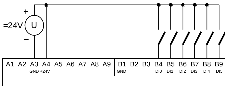
Obr.4.1 Typický příklad připojení spínačů k binárním vstupům základních modulů CP-10x5
