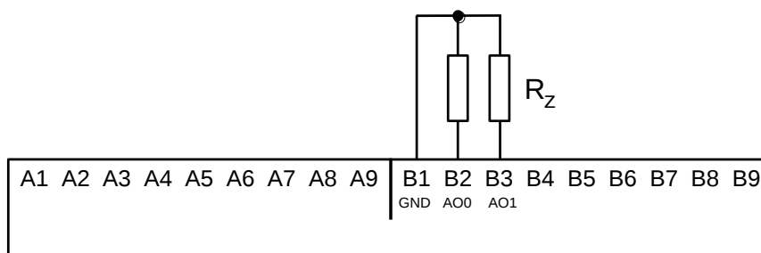
Obr.4.5 Typický příklad připojení zátěží k analogovým výstupům základních modulů CP-10x5
