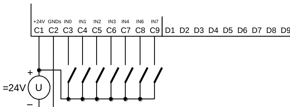
Obr.3.2 Typický příklad připojení spínačů k základnímu modulu při osazeném submodule PX-7811 na kanálu CH2
