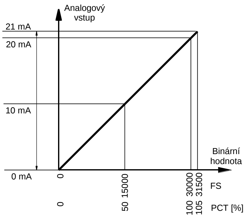
Obr.4.11 Proudový rozsah 0 až 20 mA analogových vstupů modulů CP-10x5
