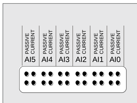
Obr.4.3 Nastavovací pole na spodní straně modulu CP-10x5 (staré provedení)
