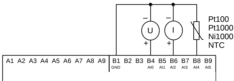
Obr.4.4 Typický příklad připojení signálů k analogovým vstupům základních modulů CP-10x5 (jednotlivé druhy signálů jsou připojitelné ke kterémukoli analogovému vstupu)
