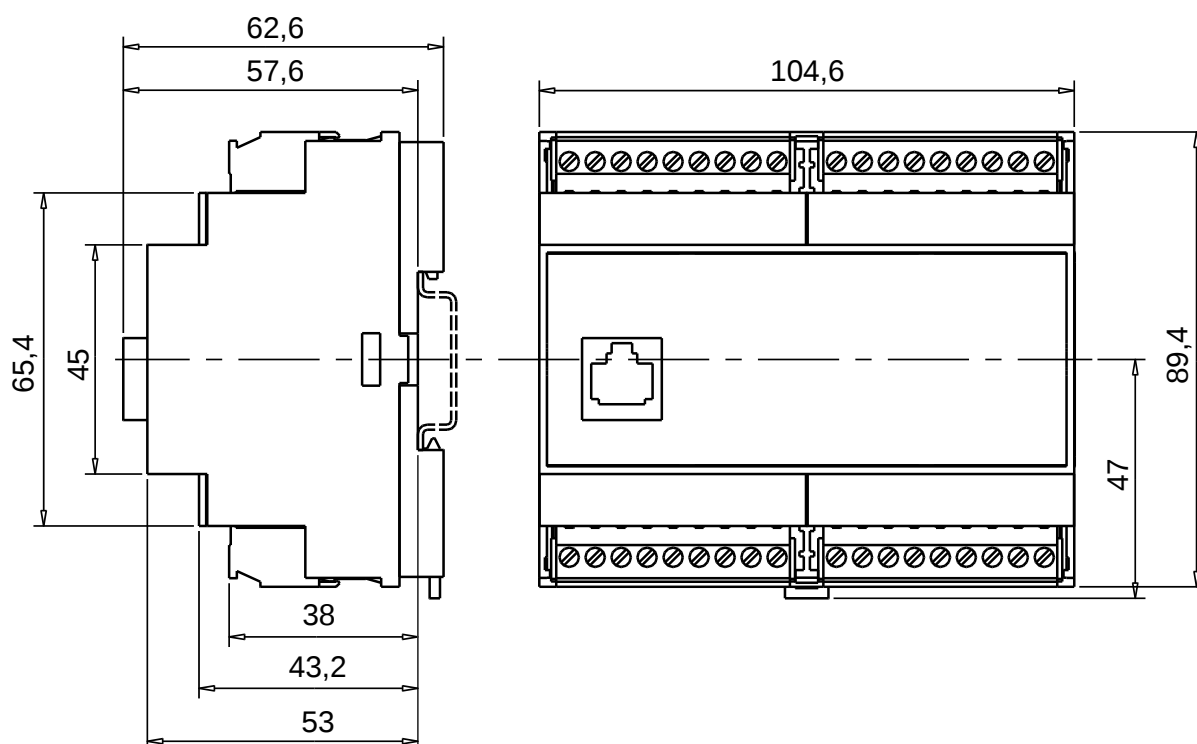
Obr.2.2 Rozměry základních modulů CP-10x5 v provedení s vyjímatelnými svorkovnicemi
