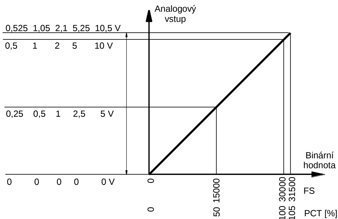
Obr.4.10 Napěťové rozsahy analogových vstupů modulů CP-10x5
