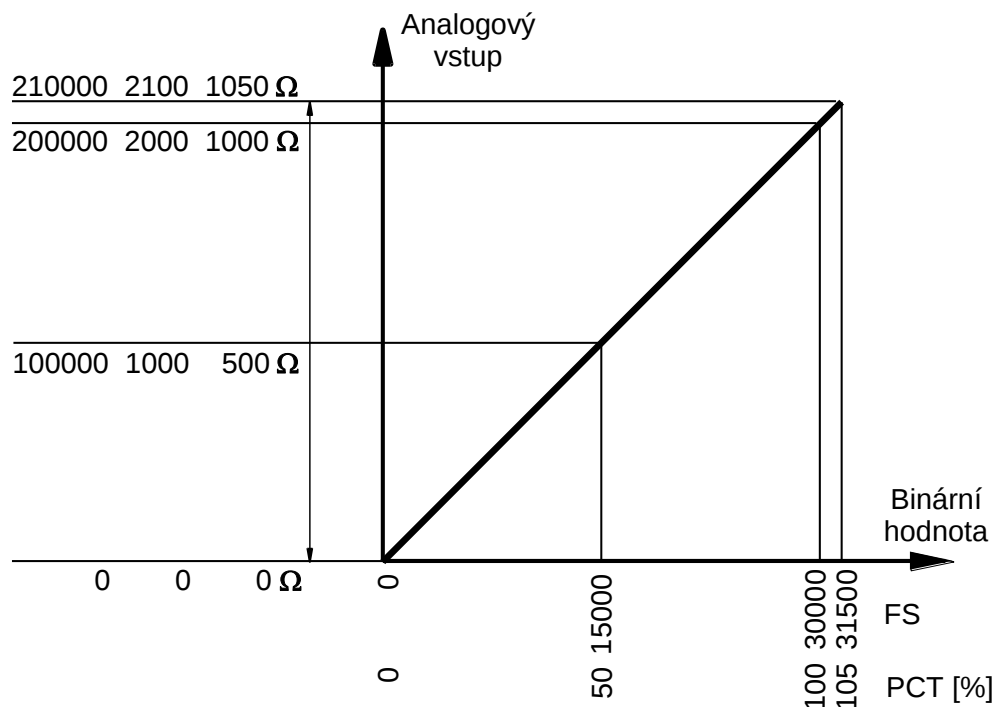
Obr.4.14 Odporové rozsahy analogových vstupů modulu CP-10x5
