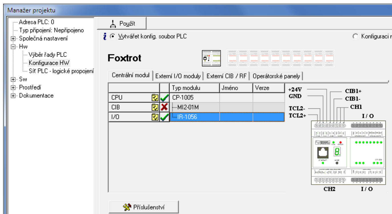
Obr.4.7 Konfigurace základního modulu CP-1005
