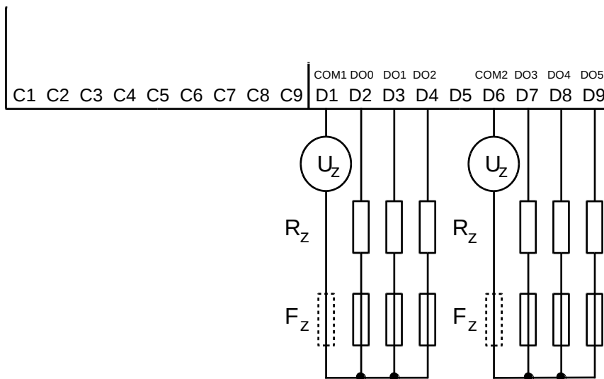
Obr.4.2 Typický příklad připojení zátěží k reléovým výstupům základních modulů CP-10x5
