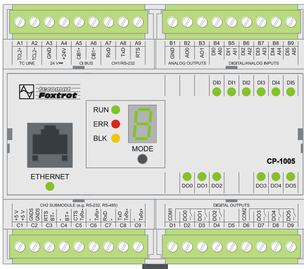
Obr.2.4 Základní modul CP-1005 - provedení od roku 2012
