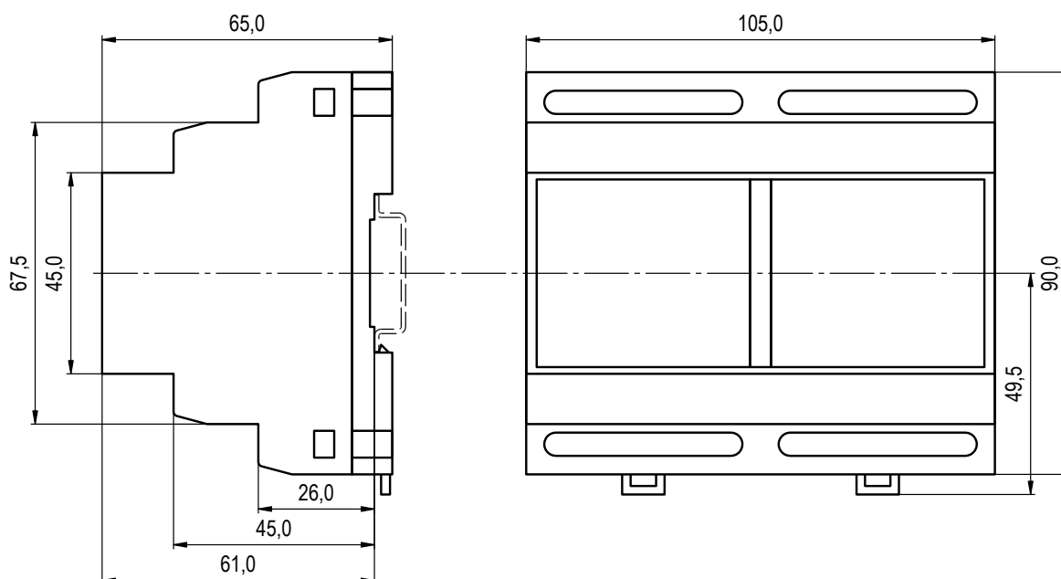
Obr.2.1 Rozměry základních modulů CP-10x5 v provedení s pevnými svorkovnicemi
