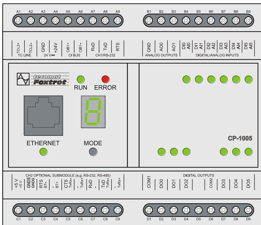
Obr.2.3 Základní modul CP-1005 - provedení do roku 2012
