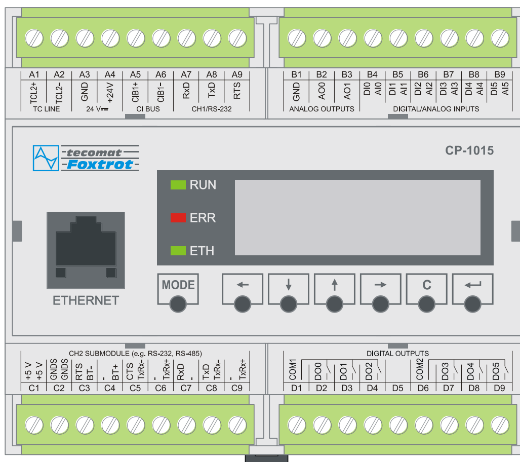
Obr.2.6 Základní modul CP-1015 - provedení od roku 2012
