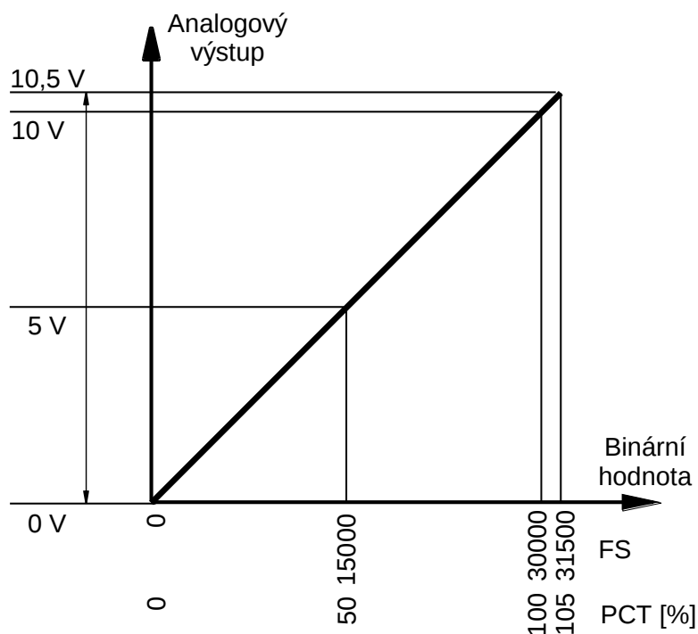
Obr.4.16 Rozsah analogových výstupů modulů CP-10x5
