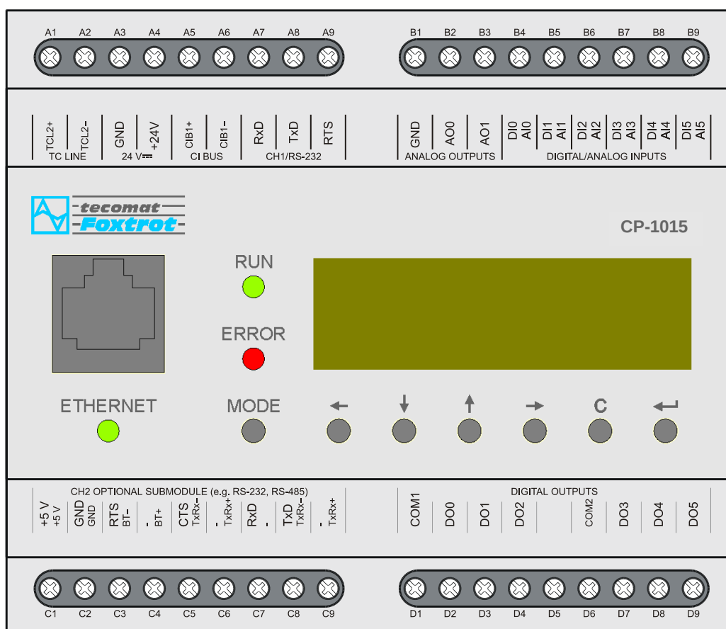
Obr.2.5 Základní modul CP-1015 - provedení do roku 2012
