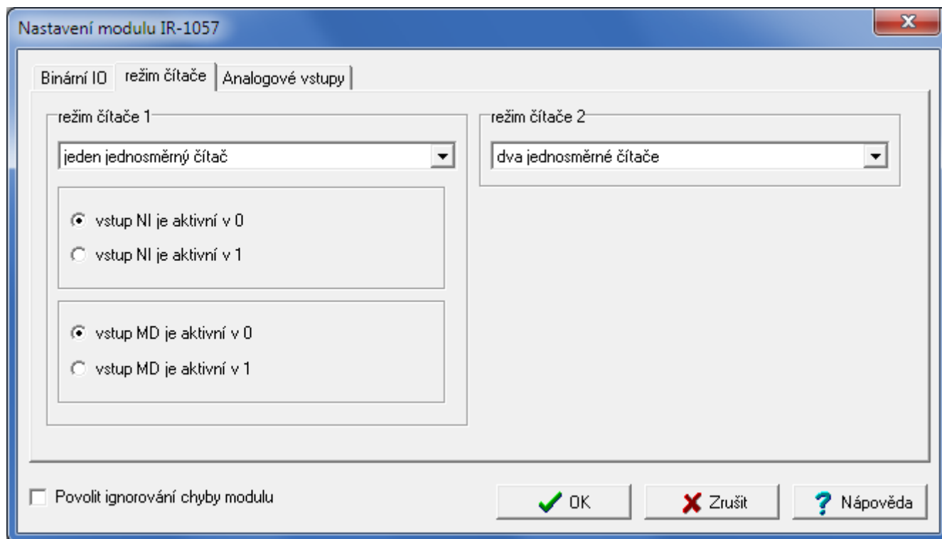
Obr.4.13 Konfigurace čítačů
