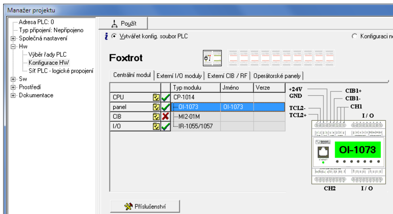
Obr.5.2 Konfigurace základního modulu CP-1014
