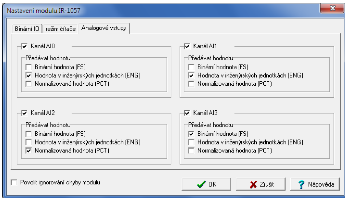
Obr.4.11 Konfigurace analogových vstupů
