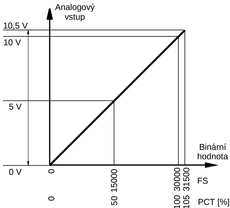
Obr.4.12 Napěťový rozsah analogových vstupů modulů CP-10x4
