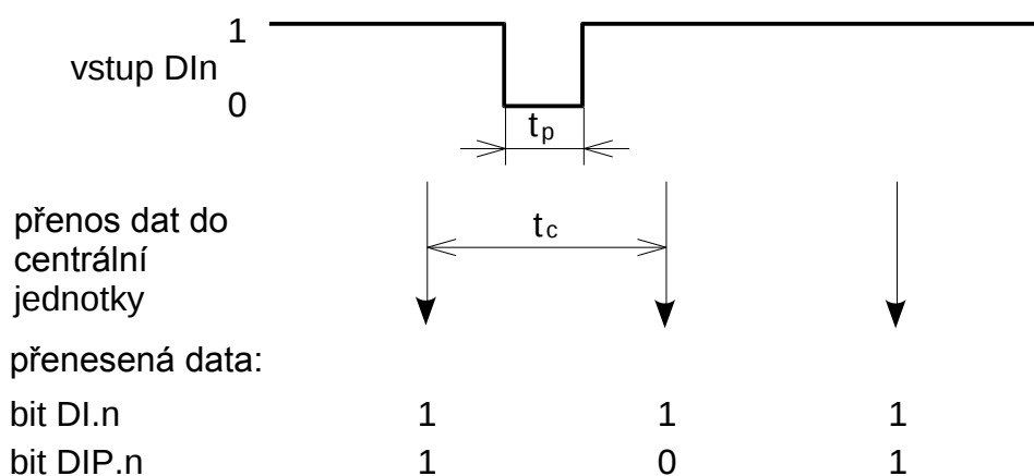
Obr.4.9 Funkce detekce krátkých pulzů do log.0 t_p - šířka pulzu, t_c = doba cyklu PLC
