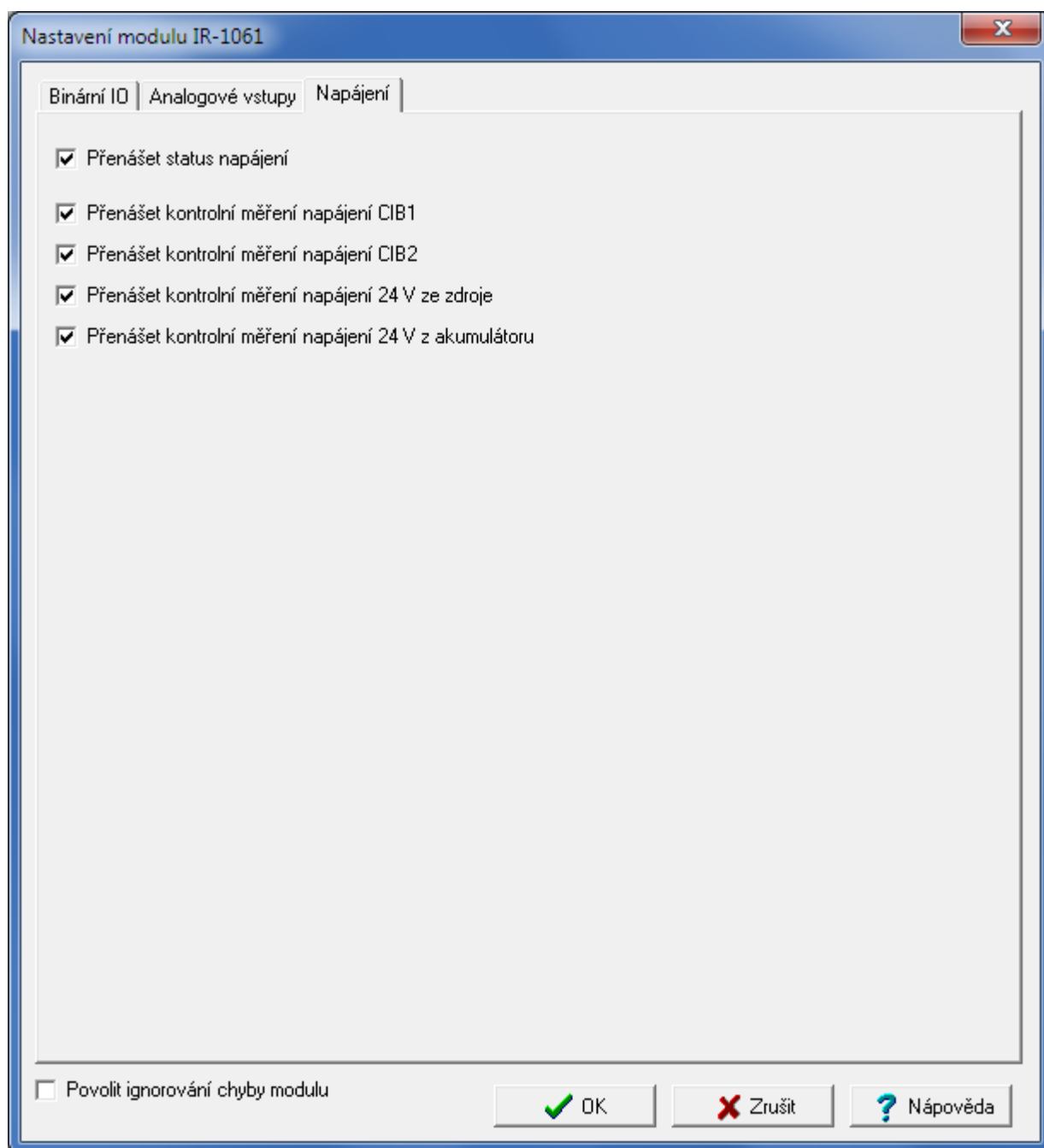
Obr.4.12 Konfigurace diagnostiky napájení
