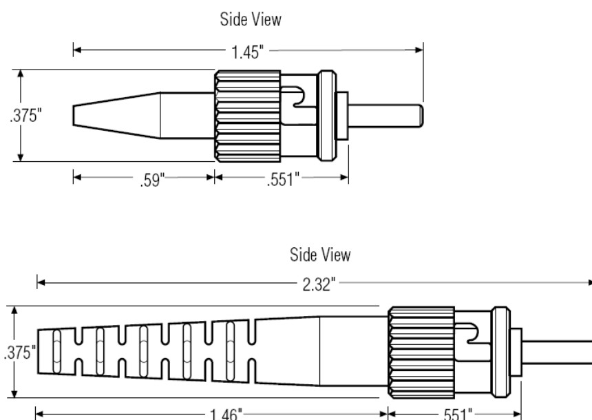
Obr.5.2 Mechanické rozměry optického konektoru ST
