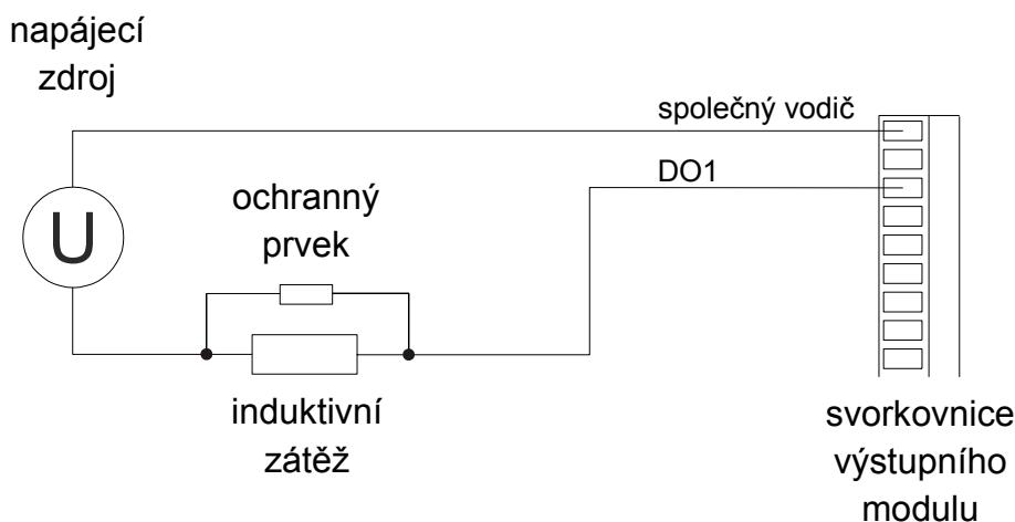
Obr.5.3 Zapojení ochranného prvku paralelně k zátěži
