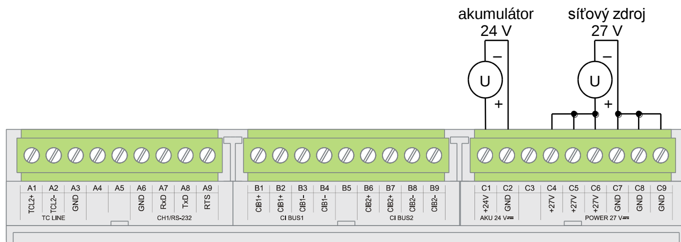
Obr.4.4 Typický příklad zapojení napájení základního modulu CP-10x0
