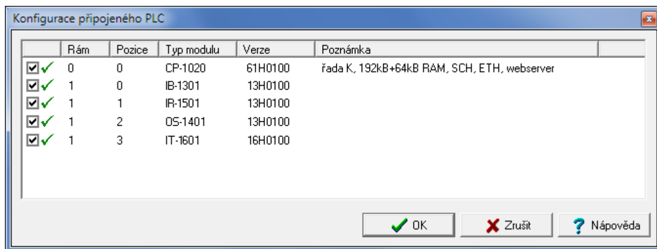
Obr.6.6 Načtení konfigurace z PLC
