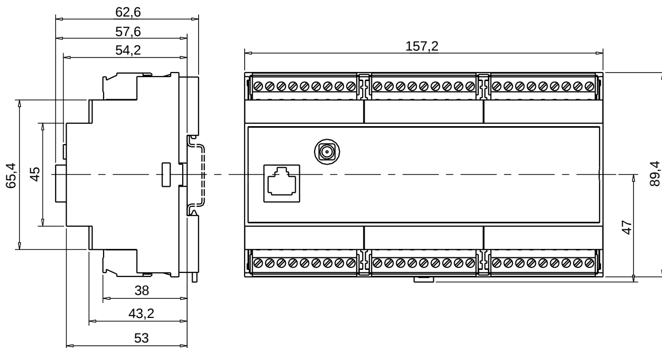
Obr.2.1 Rozměry základních modulů CP-10x0 a CP-10x1
