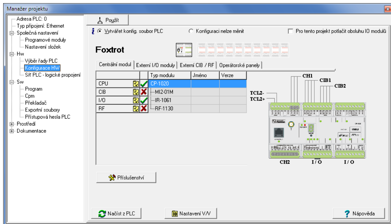
Obr.6.4 Nastavení konfigurace PLC FOXTROT - základní modul
