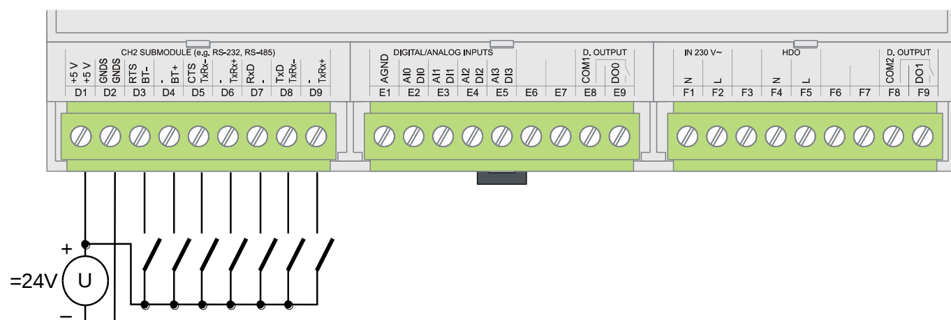
Obr.3.2 Typický příklad připojení spínačů k základnímu modulu při osazeném submodulu PX-7811 na kanálu CH2
