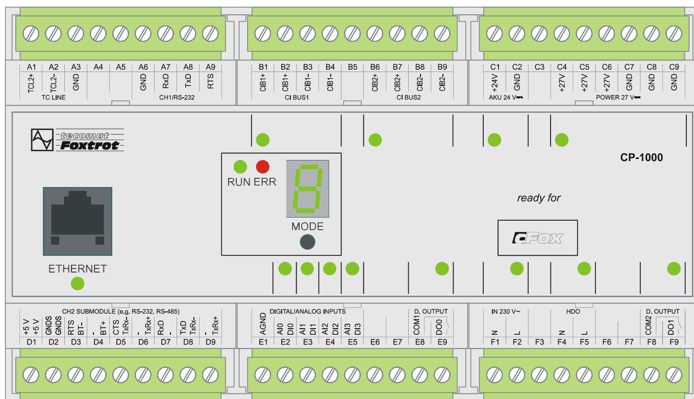
Obr.2.2 Základní modul CP-1000
