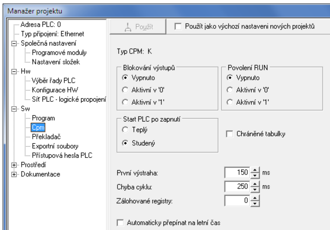
Obr.6.2 Nastavení konfiguračních konstant
