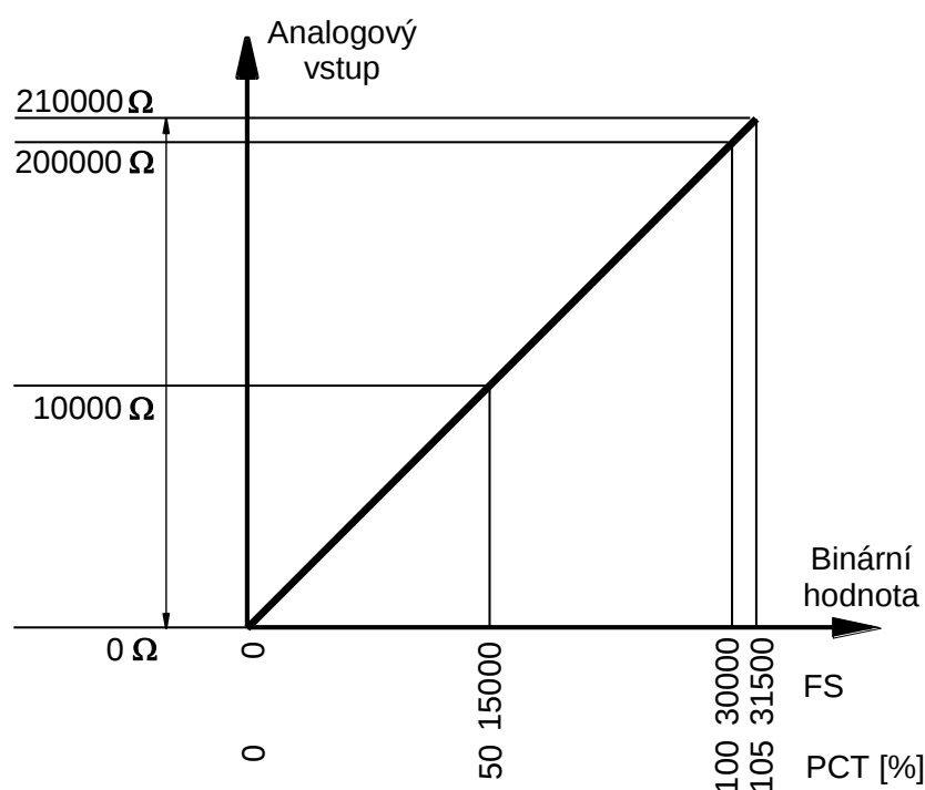
Obr.4.11 Odporový rozsah do 200 kΩ analogových vstupů modulů CP-10x0 a CP-10x1
