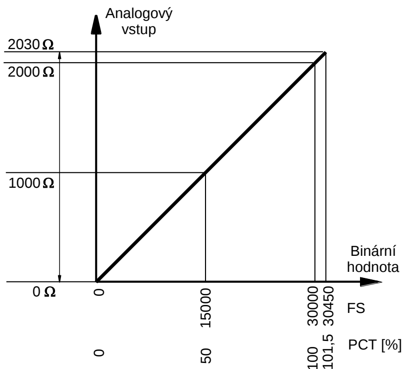
Obr.4.10 Odporový rozsah do 2000 \Omega analogových vstupů modulů CP-10x0 a CP-10x1 (rozsah je v oblasti nad nominální hodnotou zkrácen z důvodu fyzického omezení rozsahu vstupů)
