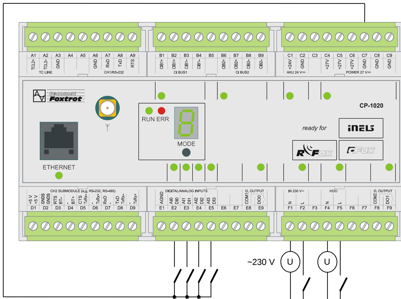
Obr.4.1 Typický příklad připojení spínačů k binárním vstupům základních modulů CP-10x0 a CP-10x1
