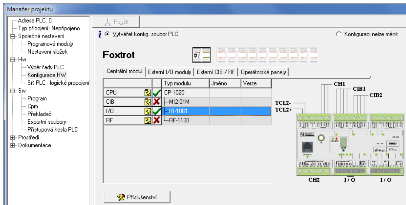
Obr.4.6 Konfigurace základního modulu CP-1020
