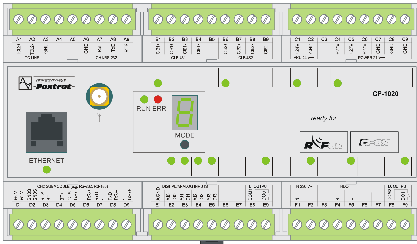
Obr.2.4 Základní modul CP-1020
