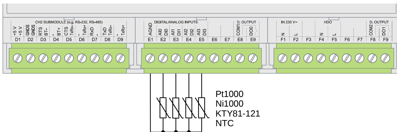
Obr.4.3 Typický příklad připojení signálů k analogovým vstupům základních modulů CP-10x0 a CP-10x1
