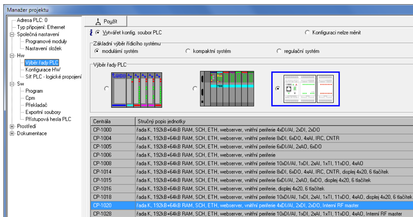
Obr.6.3 Výběr řady PLC
