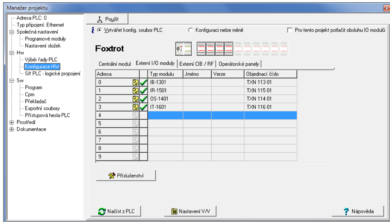
Obr.6.5 Nastavení konfigurace PLC FOXTROT - periferní moduly
