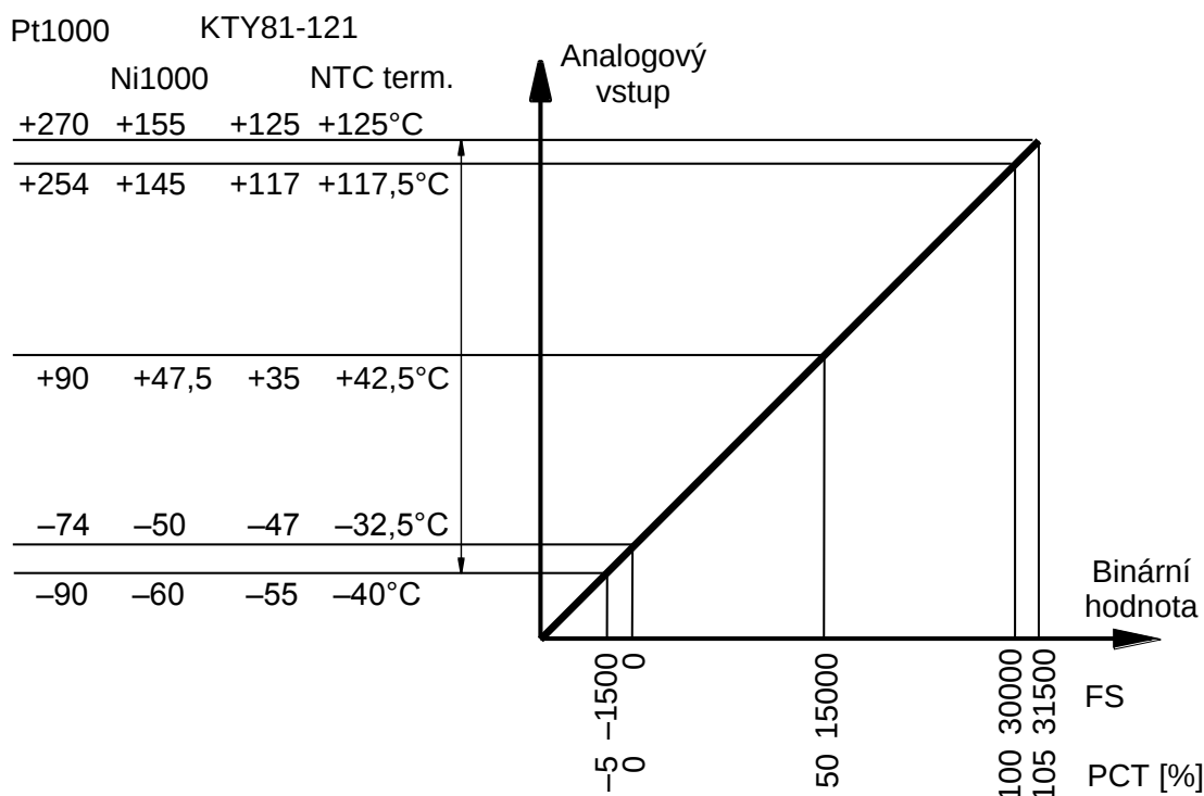
Obr.4.9 Rozsah analogových vstupů modulů CP-10x0 a CP-10x1 pro odporová čidla Pt1000, Ni1000, KTY81-121 a NTC termistory
