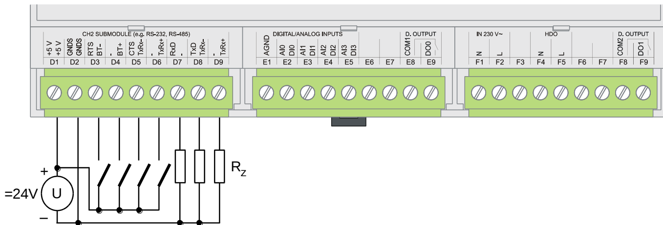
Obr.3.3 Typický příklad připojení spínačů a zátěží k základnímu modulu při osazeném submodulu PX-7812 na kanálu CH2
