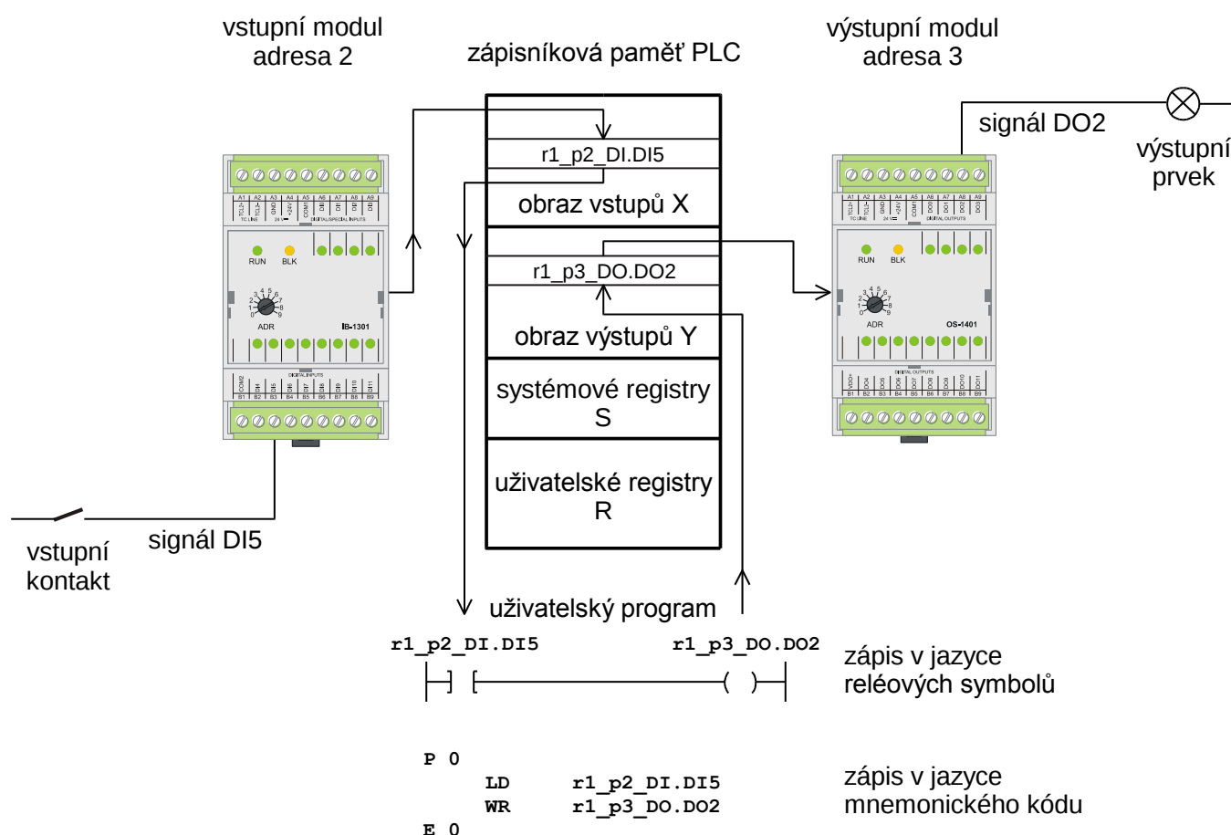
Obr.1.2 Schéma zpracování signálů programovatelným automatem (symbolická jména signálů jsou automaticky generována prostředím Mosaic, uživatel má možnost je změnit)
