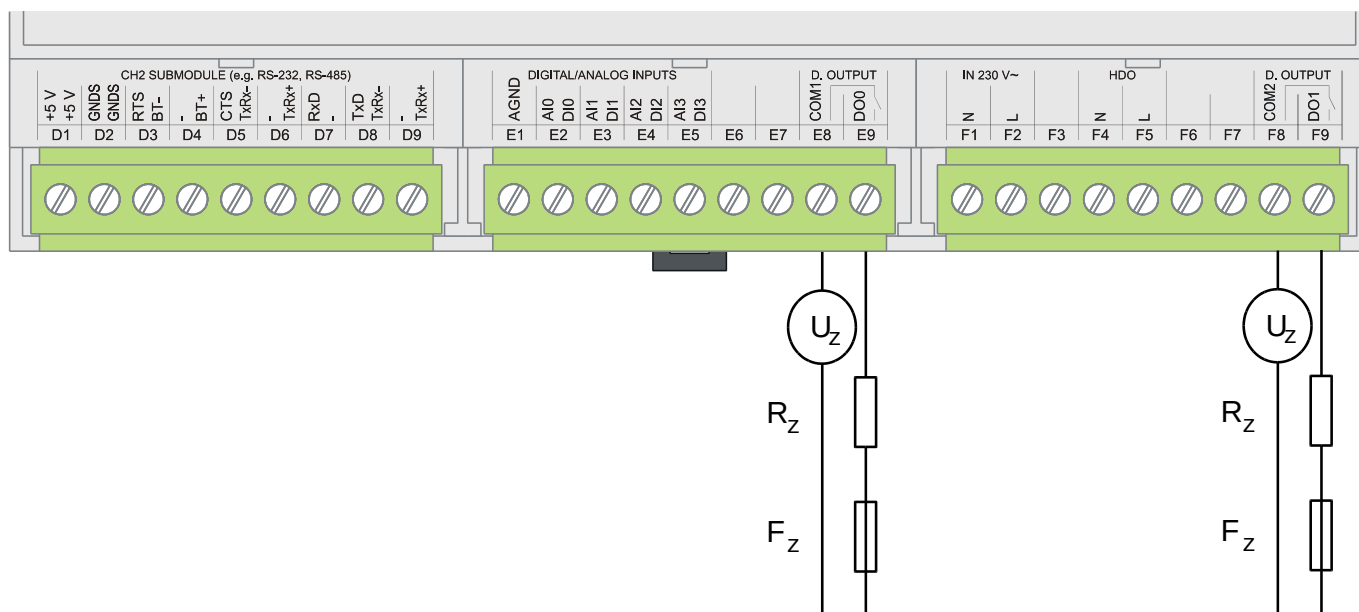
Obr.4.2 Typický příklad připojení zátěží k binárním výstupům základních modulů CP-10x0 a CP-10x1
