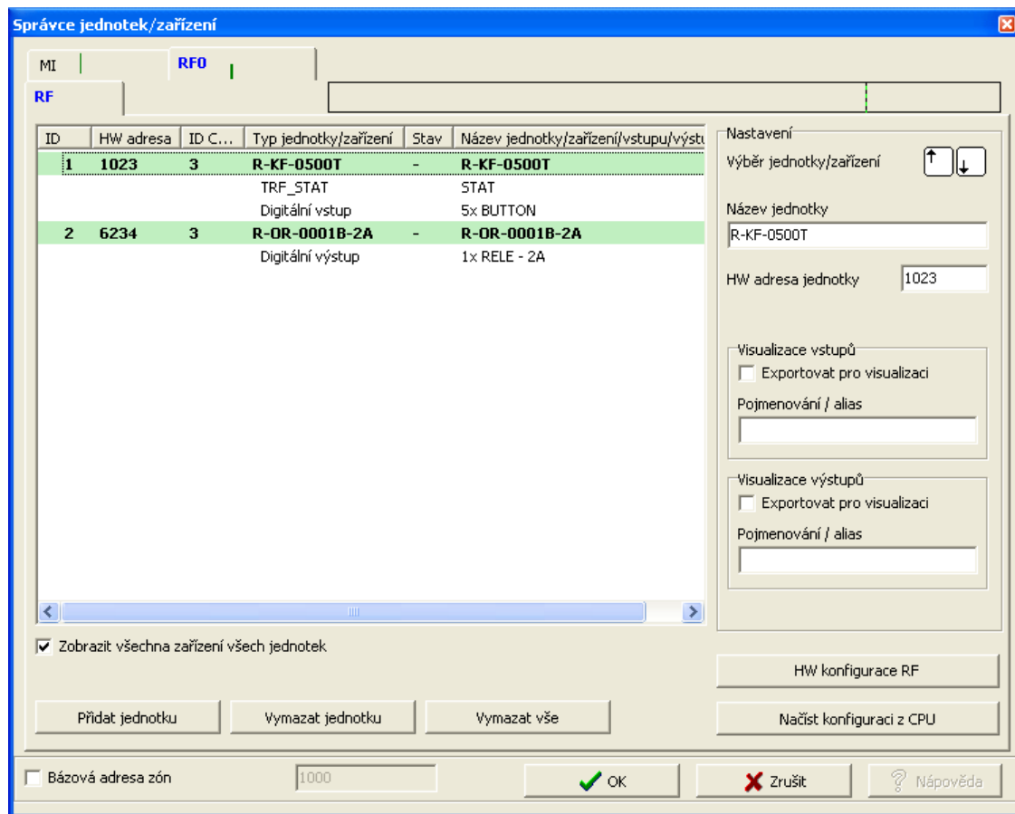
Obr. 2.5 SW konfigurace RF mastera
