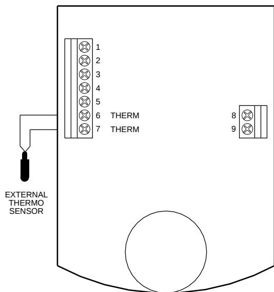
Obr. 3.26 Příklad zapojení
