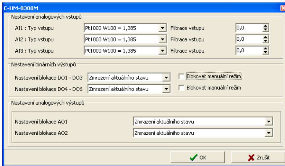
Fig. 3.5 Module configuration
