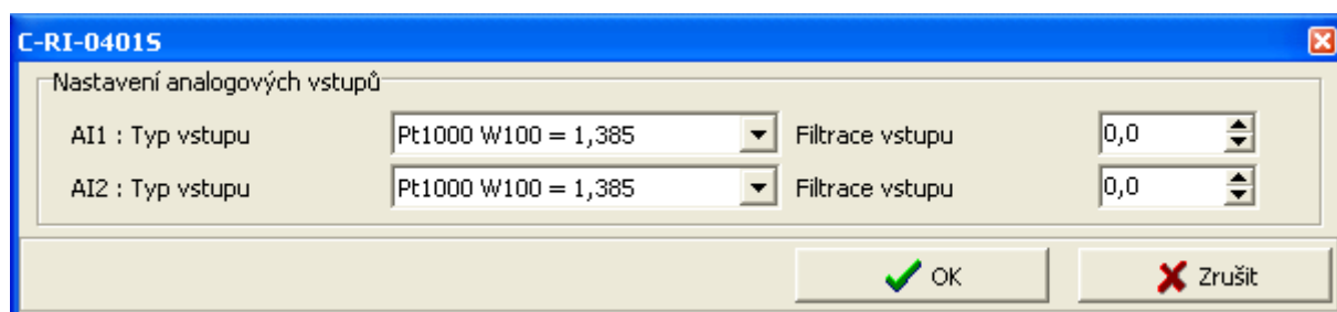
Fig. 3.75 Module configuration
